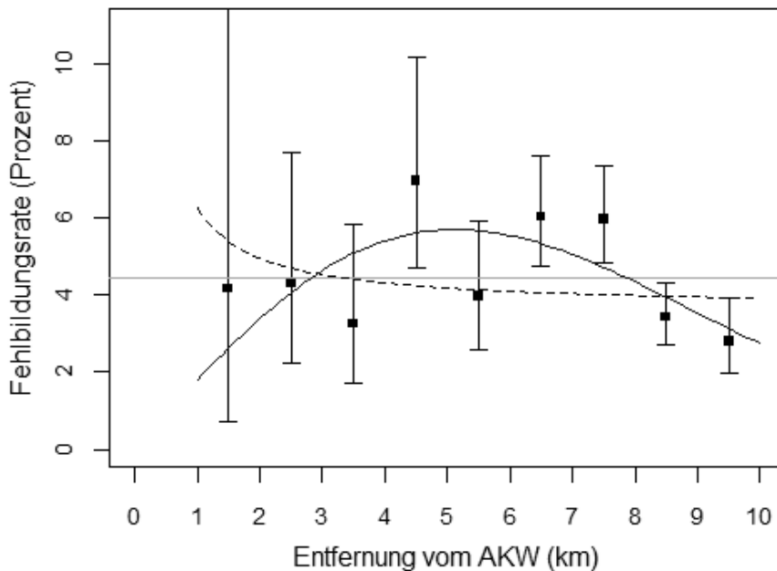
Abbildung 5: Fehlbildungsrate in der Umgebung der AKW Philippsburg und Biblis im Zeitraum 2006-2008 in Abhängigkeit von der Entfernung und Ergebnis einer Regression mit einer Rayleighfunktion für die Abstandsabhängigkeit (Körblein 2010). Die horizontale Linie zeigt den Mittelwert in der Studienregion, die gestrichelte Linie das Ergebnis einer Regression mit einem reziproken Abstandsmodell (Rate nimmt ab mit der Entfernung).
