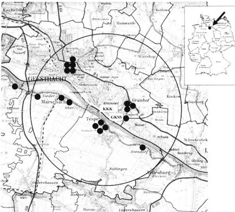
Abbildung 1: Karte zur Lokalisation von 16 Fällen mit Akuter Leukämie bei Kindern unter 15 Jahren im 5 km-Umkreis des Atomkraftwerks Krümmel (KKK) 1990-2006 Zusätzlich eingetragen: 1 Fall von 2004 „geringfügig außerhalb des Kreises“, 1 Fall eines Jugendlichen (21 Jahre, 1991), 1 kindlicher Fall Aplastische Anämie 1989 (strahleninduzierbare Blutkrankheit). (BI gegen Leukämie Elbmarsch 2006)
